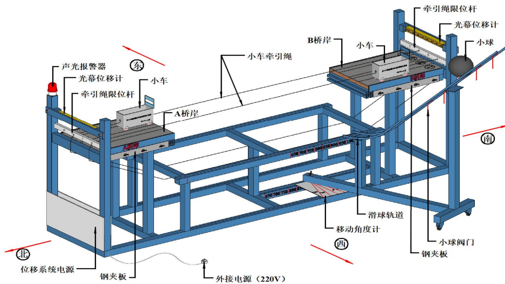
图 6 加载装置轴测示意图
