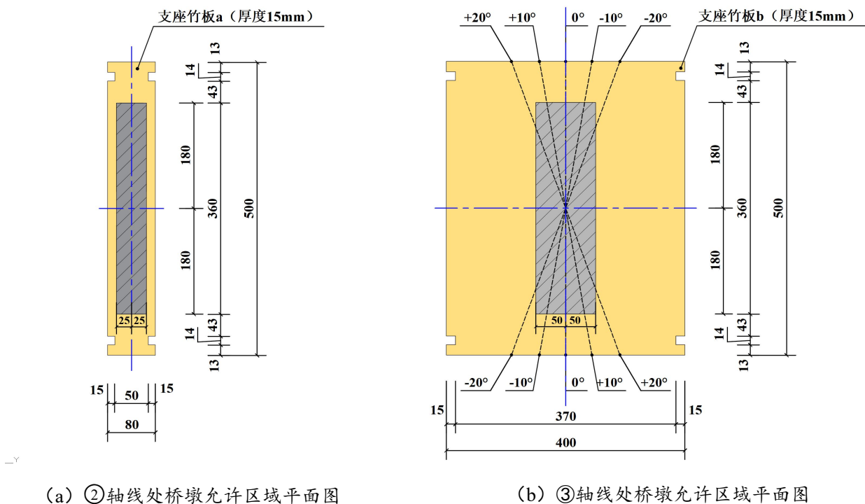
图 3 桥墩允许区域平面图（单位：mm）
