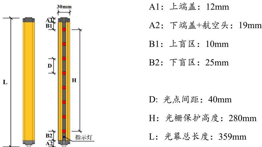
图9 光幕位移计示意图
